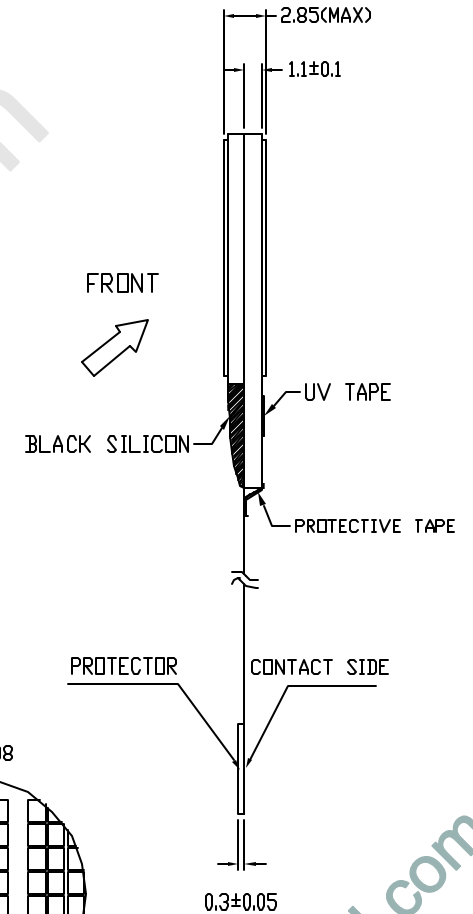
DETAIL A:
