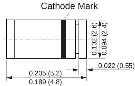
Glass MELF
