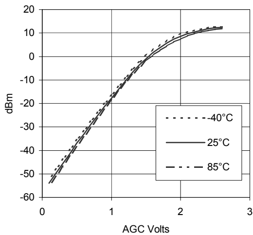
IS136 Tx. 900 MHz - Power Out v AGC (Temp.)
