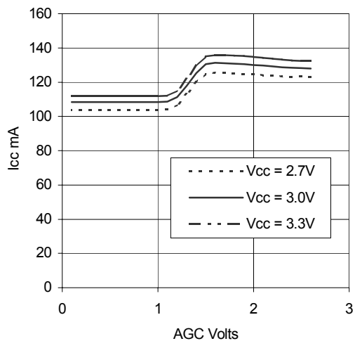
IS136 Tx. 1900 MHz - I_{cc} v AGC ( V_{cc} )
