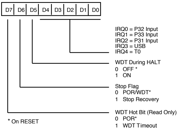
R250 IRQ
