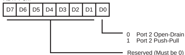
R247 P3M
