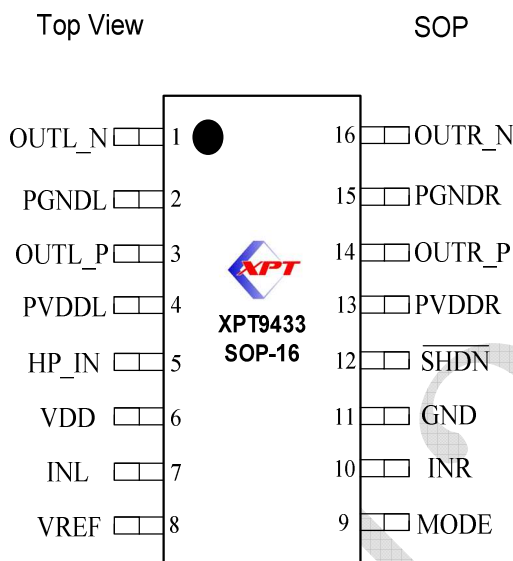
XPT9433 SOP-16 管脚分布图
