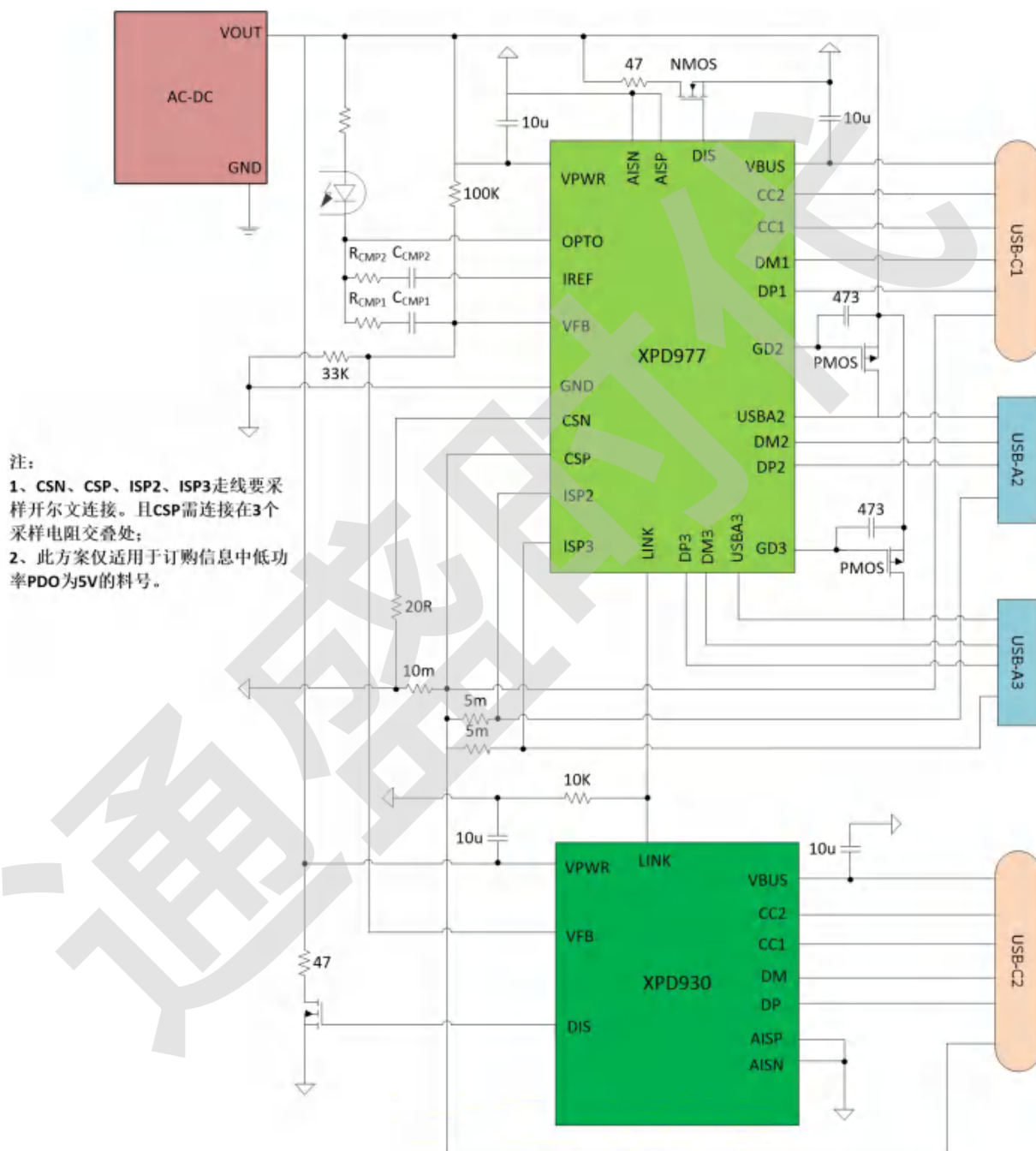
XPD977_2A+2C应用电路图
