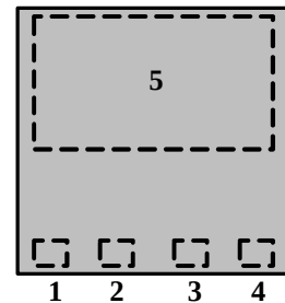
PDFN 8X8_HV
