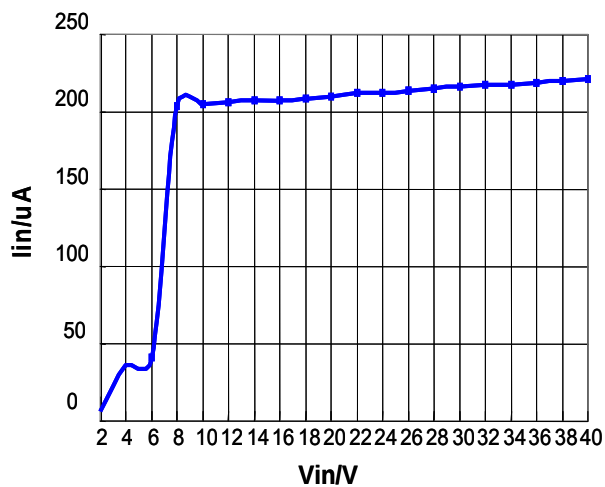
Iin vs VIN
