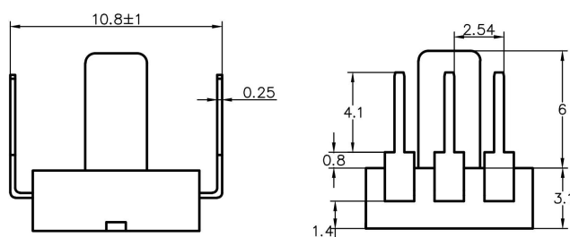
DIP-F
