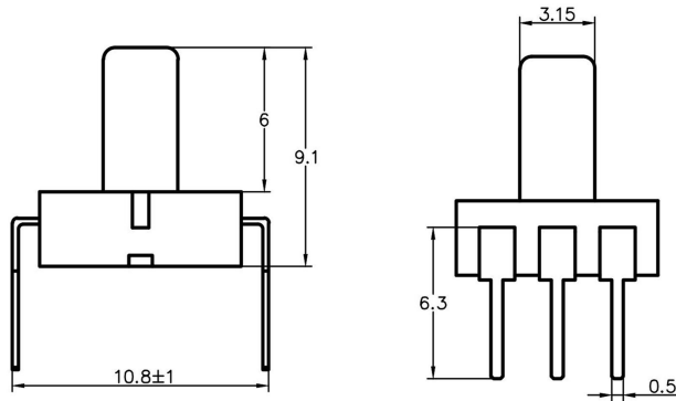
DIP-R
