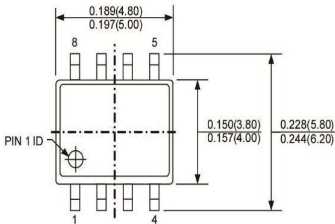
俯视图
