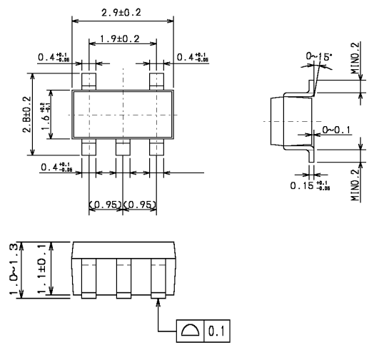
SOT-25
