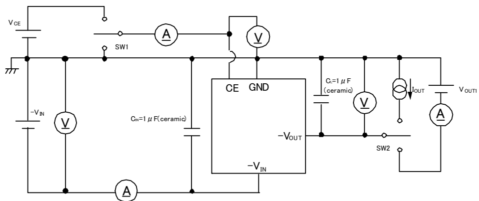
2) CIRCUIT②
