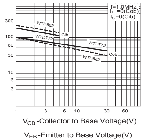
F10. C_{ob} - V_{CB} , C_{ib} - V_{CE}
