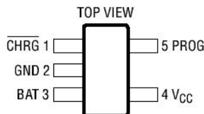
SOT23-5 封装
