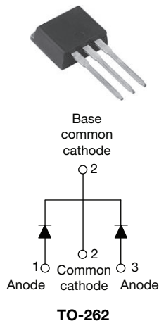
VS-10CTQ150-1PbF
