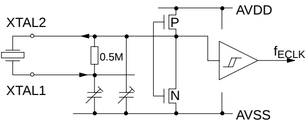
Fig. 3-8: Crystal Oscillator
