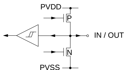
Fig. 6-9: Input/Output PIXCLK
