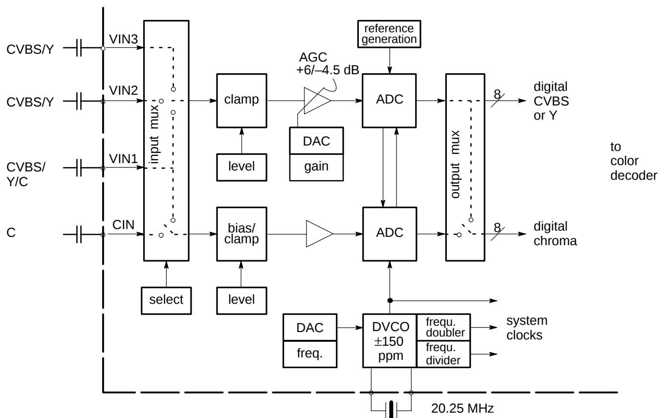
Fig. 2–2: Analog front-end
