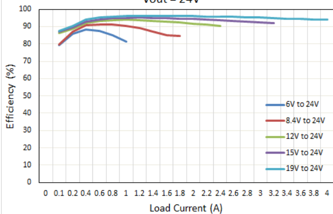
Vout = 24V
