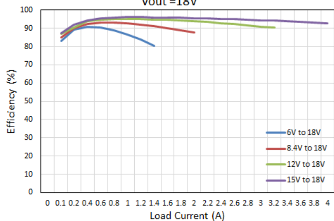
Vout = 18V
