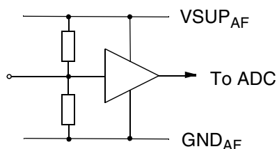
Fig. 6-10: Input pins CIN1, CIN2
