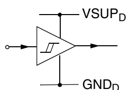
Fig. 6-31: Input pins VB0-VB7, VBCLK
