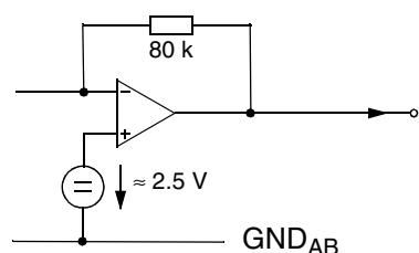
Fig. 6-26: Output pins AOUT1, AOUT2
