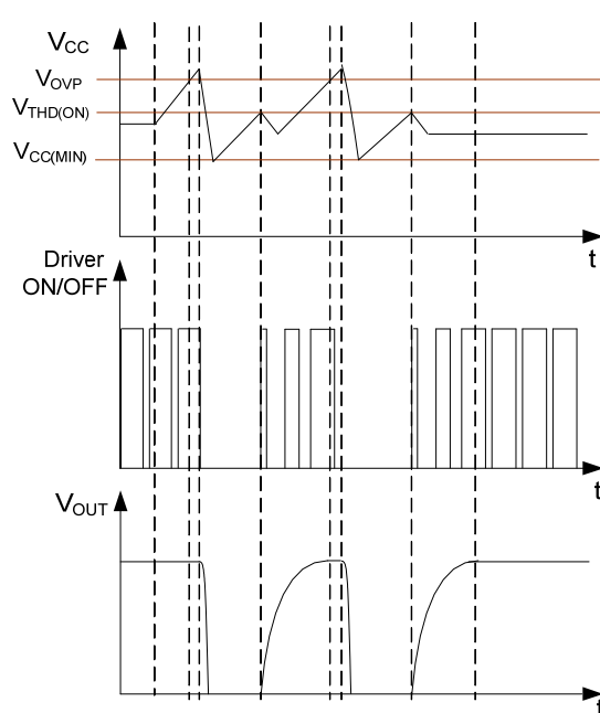
Fig.7 OVP case
