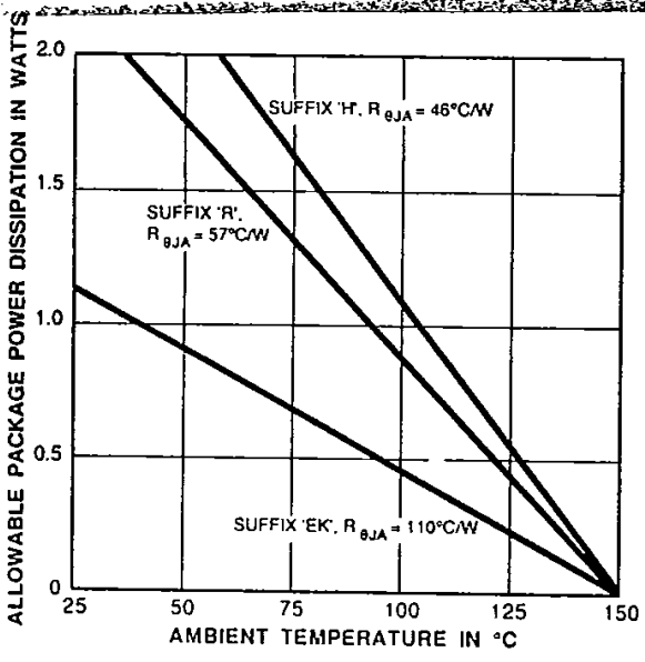
Dwg. GM-004
