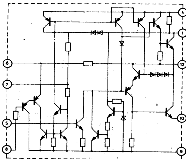
Schemat wewnętrzny
