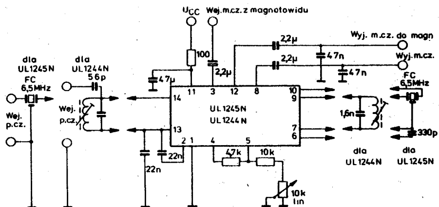
Schemat aplikacyjny
