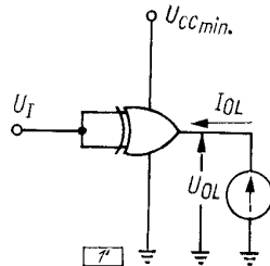
Układ pomiarowy 1'
