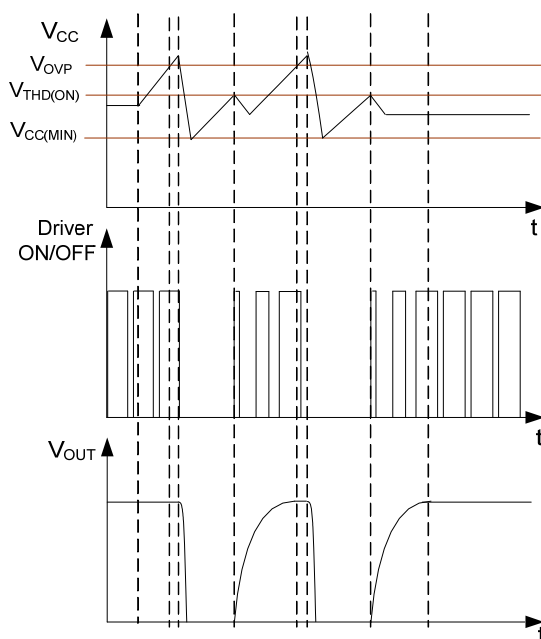
Fig.6 OVP case
