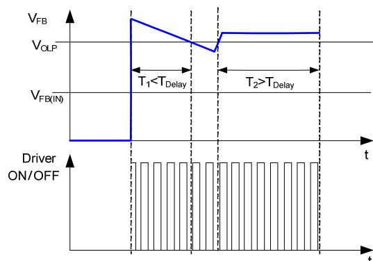
Fig.4 OLP case
