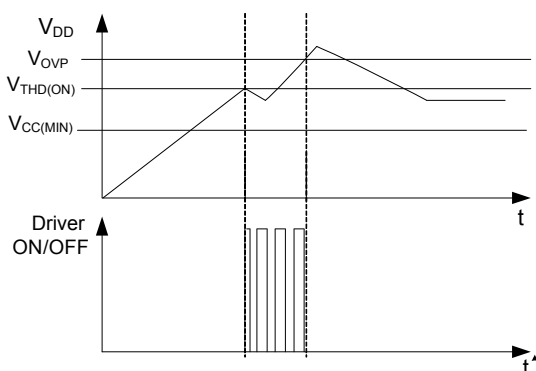
Fig.3 OVP case
