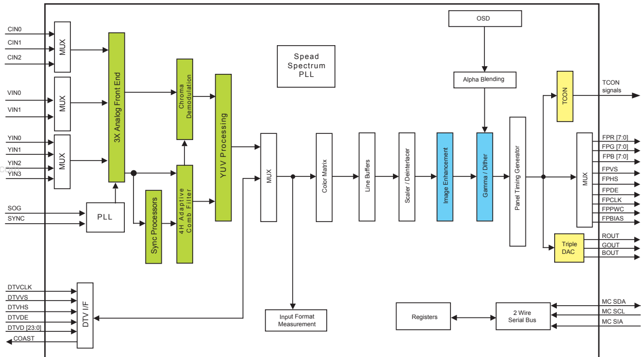
TW8806 / TW8807 Block Diagram
