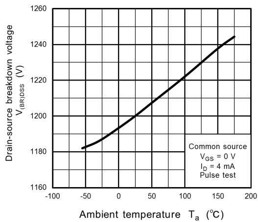
Fig. 8.11 V_{DS} - T_a
