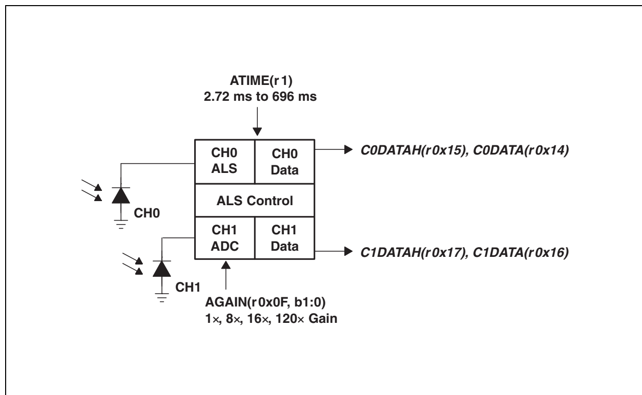
Figure 16: ALS Operation
