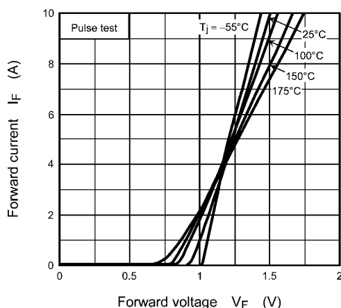
Fig. 9.1 I_F - V_F
