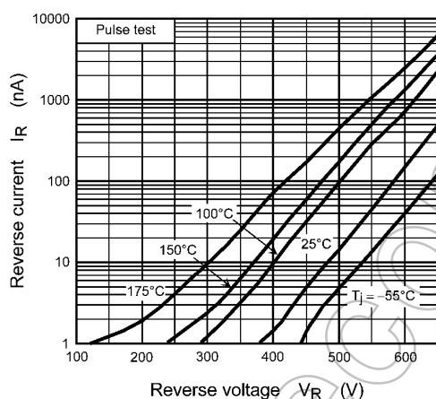
Fig. 9.3 I_R - V_R
