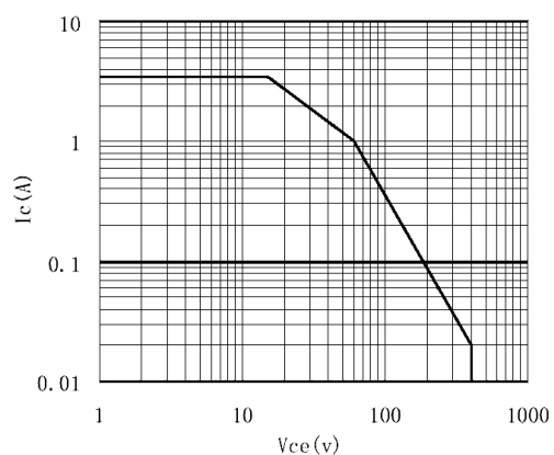
Vces - Ic
