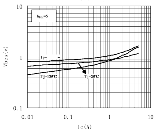
Vbes - Ic
