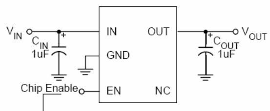
SOT23 - 5
