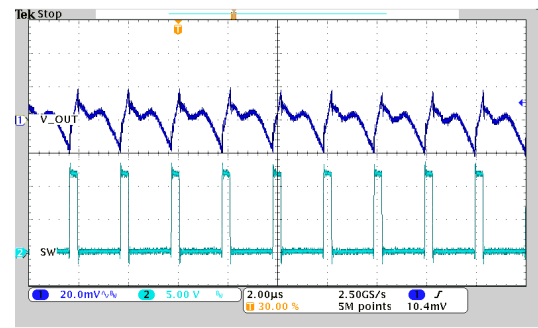
DC Ripple
