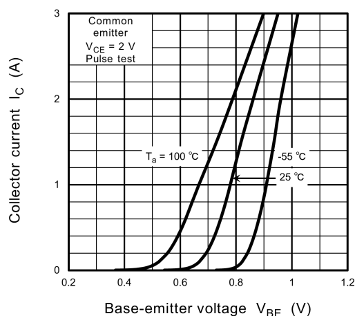
Fig. 7.5 I_C - V_{BE}
