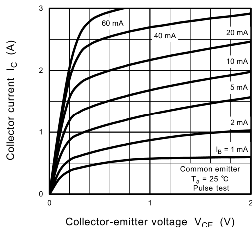
Fig. 7.1 I_C - V_{CE}
