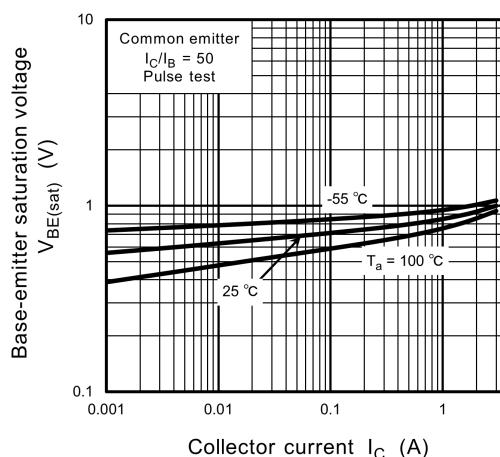
Fig. 7.4 V_{BE(sat)} - I_C
