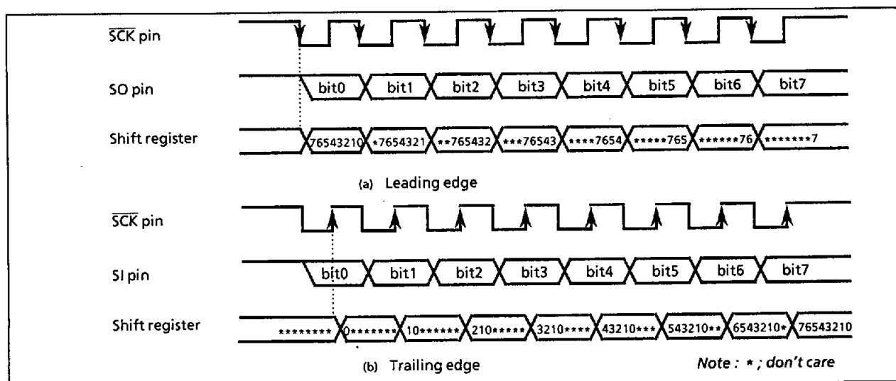
Figure 2-52. Shift Edge
