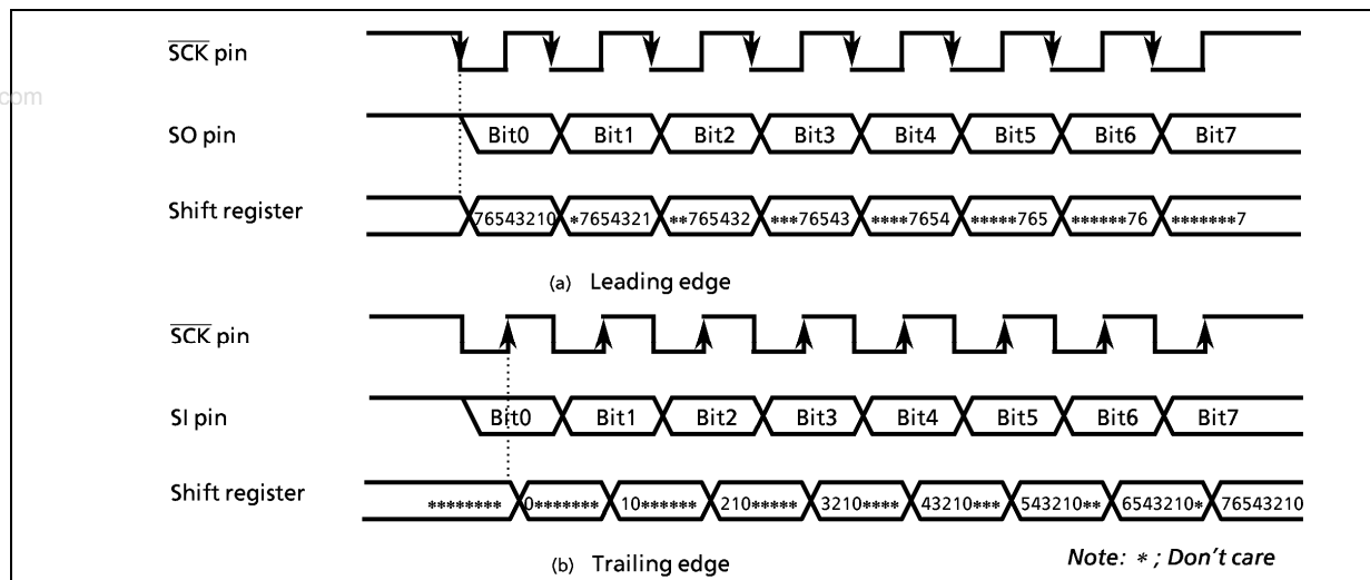
Figure 2-41. Shift edge
