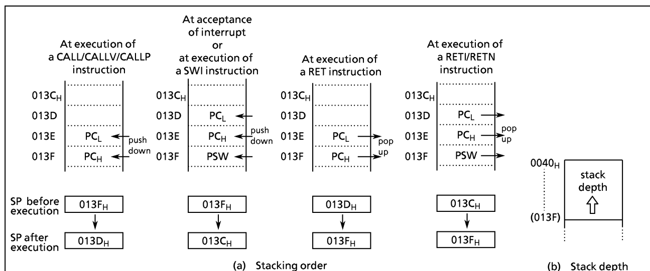
Figure 1-8. Stack
