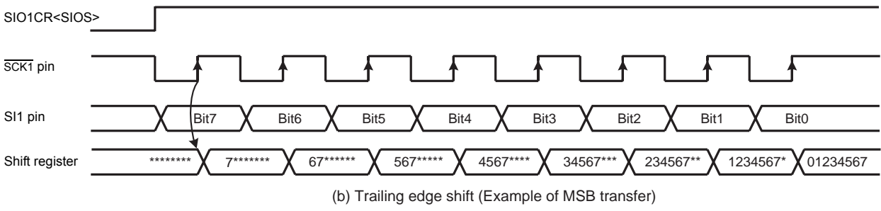
Figure 14-4 Shift Edge
