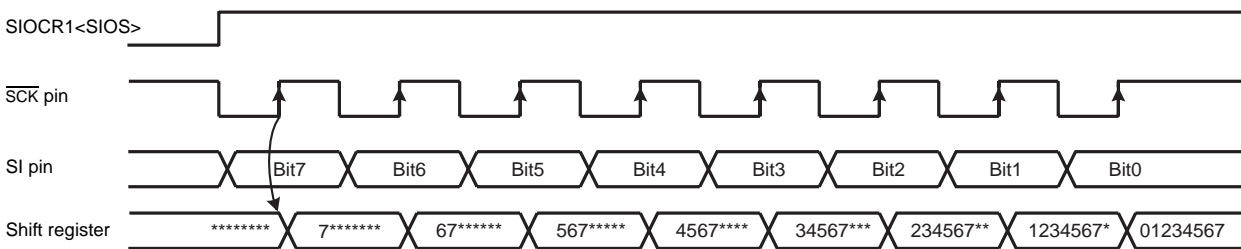
Figure 10-4 Shift Edge
