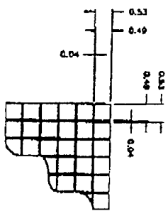
DETAIL A:
