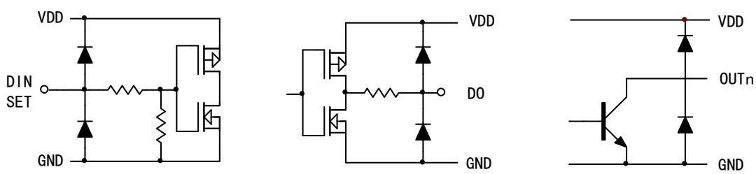
输出及输入等效电路
