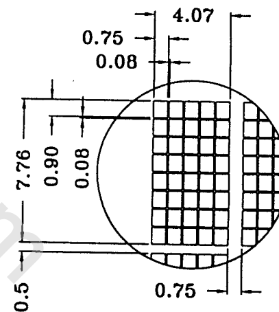
DETIAL A:
