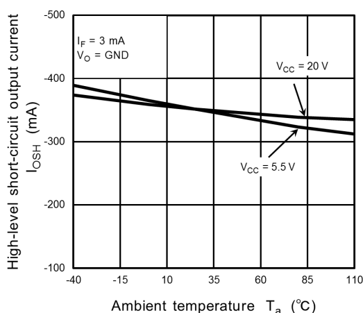
Fig. 13.2.10 I_{OH} - T_a
