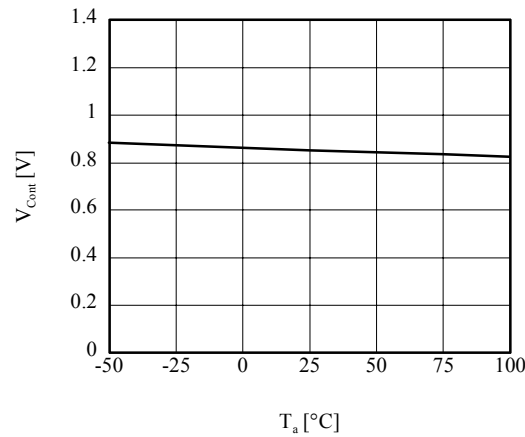
■ V_{Cont} vs T_a (TK63128B/H/S)
