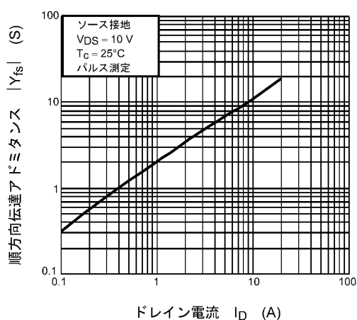
図 8.5 |Y_{fs}| - I_D
