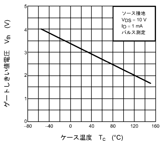
図 8.10 V_{th} - T_C
