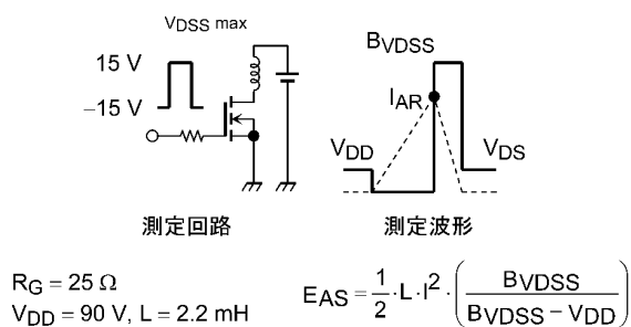
図 8.16 測定回路/測定波形
