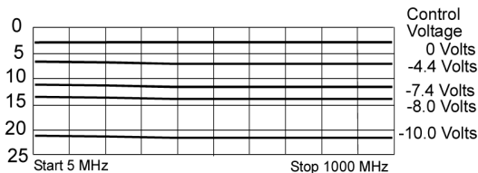
Attenuation
