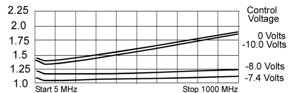
Output VSWR
