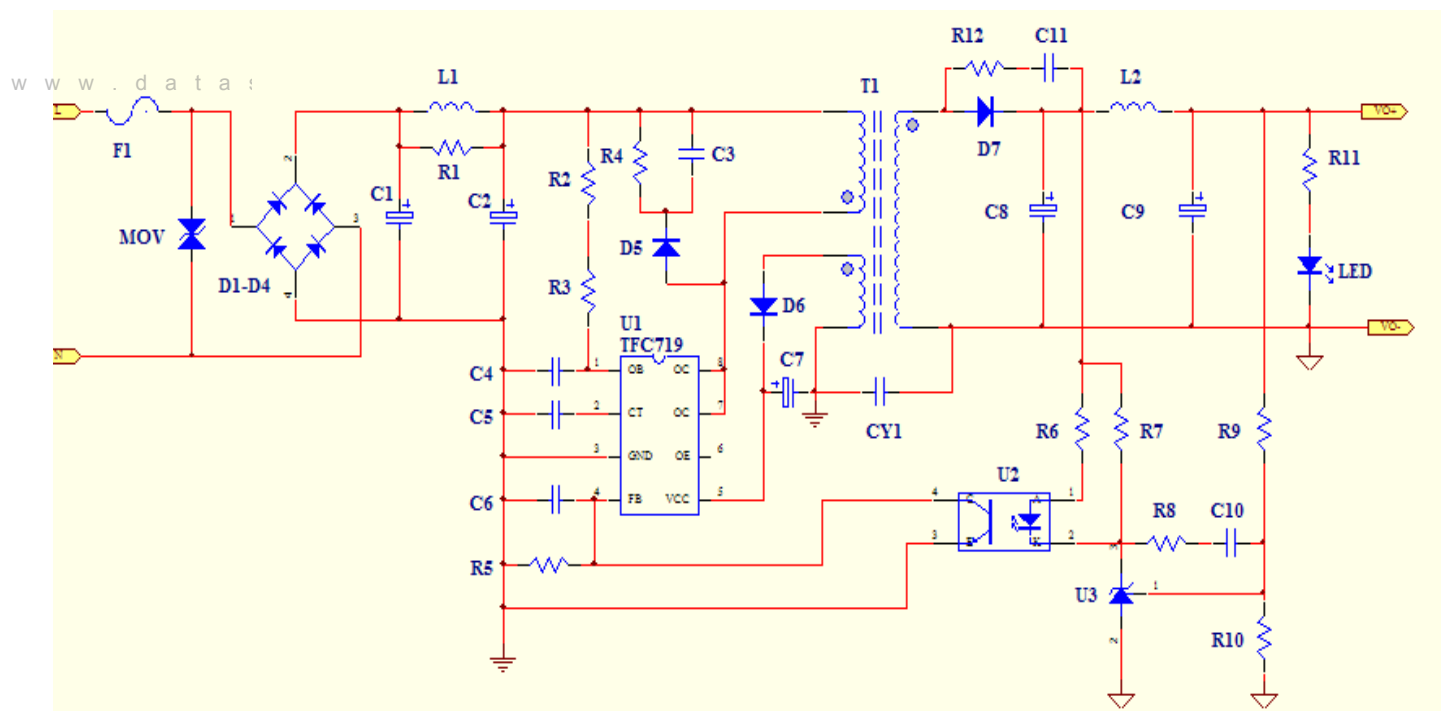
图10. 典型应用电路
