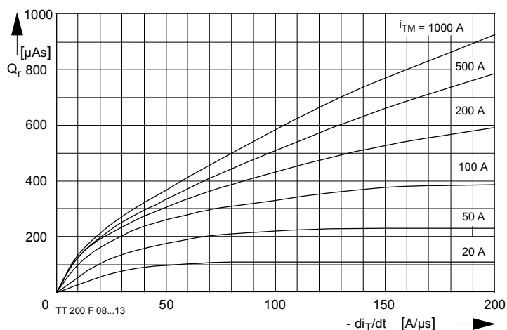
Bild / Fig. 17 Sperrverzögerungsladung Q_r = f(di/dt) t_{vj} = t_{vj \text{ max}}, v_R = 0,5 V_{RRM}, v_{RM} = 0,8 V_{RRM} Parameter: Durchlaßstrom i_{TM} Recover charge Q_r = f(di/dt) t_{vj} = t_{vj \text{ max}}, v_R = 0,5 V_{RRM}, v_{RM} = 0,8 V_{RRM} Parameter: on-state current i_{TM}
