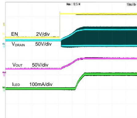
Startup from EN
