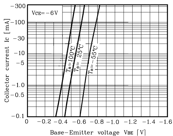
Fig. 1 I_C - V_{BE}
